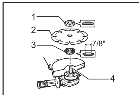
► 1. Contre-écrou 2. Meule diamantée 3. Bague interne 4. Axe
