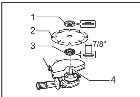
► 1. Contratuercas 2. Disco de diamante 3. Brida interior 4. Eje
