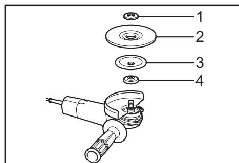
► 1. Contre-écrou 2. Meule flexible 3. Tampon d'ap-point 4. Bague interne
